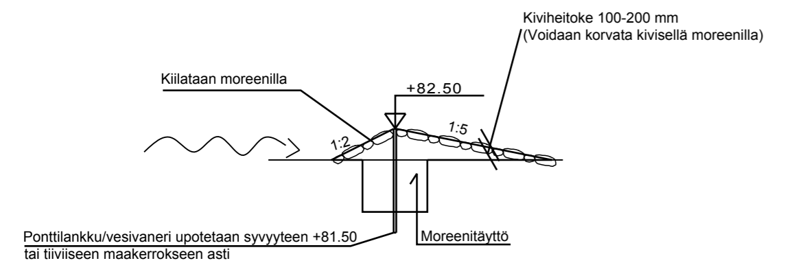
Pohjapadon A periaatepiirustus
