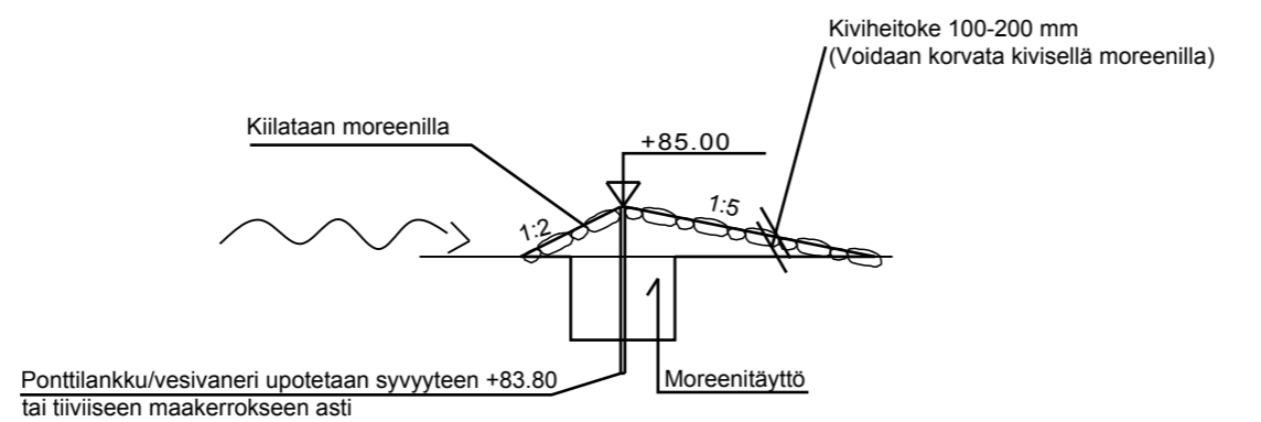
Pohjapadon B periaatepiirustus
